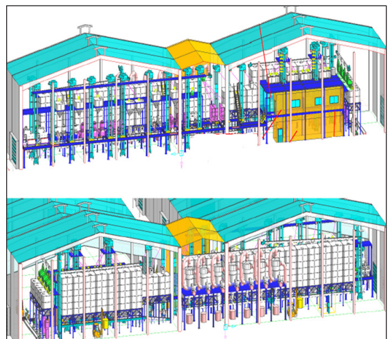
တွံတေးတွင် တပ်ဆင်တည်ဆောက်မည့် Rice Mill ပုံစံ
