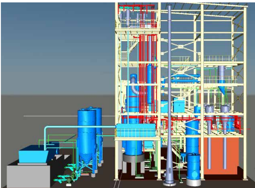
ဆီချောထုတ်စက်ရုံ၏ အတွင်းတည်ဆောက်ပုံ
